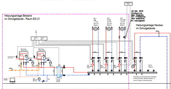
Schule - Bestand
