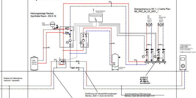
Sporthalle - Neubau
